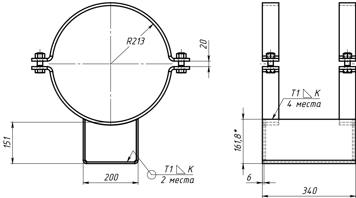
Поз.3 (Полухомут)
