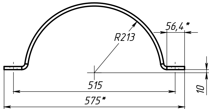
Поз.3 (Полухомут)
