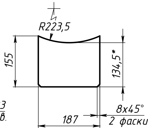
Поз.2 (Ребро)
